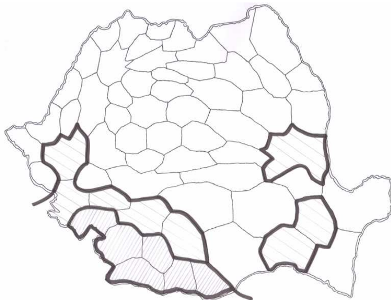
Abb. 4. Areale Verteilung von Übernahmen aus den nebulgarischen Mundarten im Rumänischen auf den Karten des ALR II S. n., cf. in Leschber (2005c) aximum der Lexeme entspricht 100 % des bisher festgestellten Vorkommens auf einem Erhebungspunkt Markierung 100 % - 75 % des Vorkommens (dichte Schraffur) Markierung 75 % - 50 % des Vorkommens (weite Schraffur)
